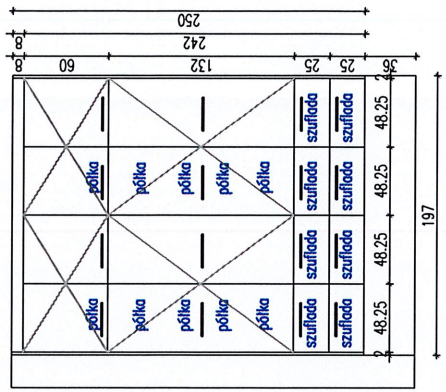
WIDOK ŚCIANY 3
