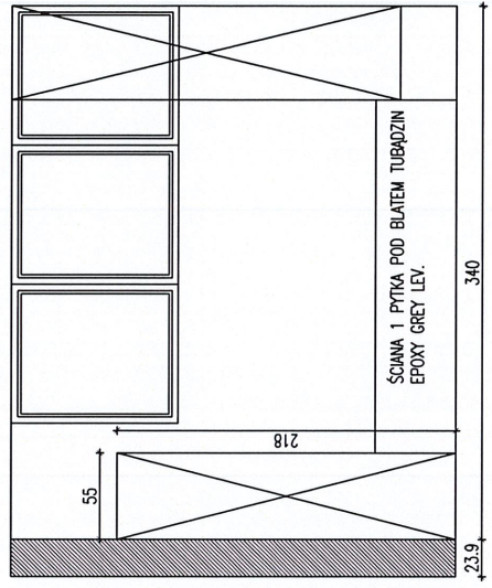
WIDOK ŚCIANY 2
