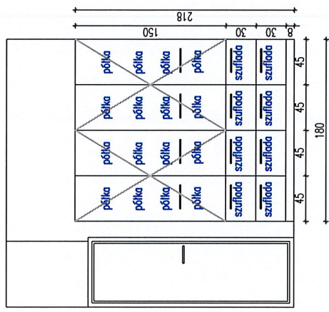
WIDOK ŚCIANY 1
