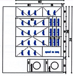
WIDOK SCIANY 6
