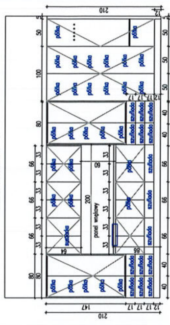
WIDOK ŚCIANY 1
