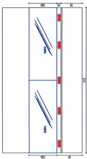
WIDOK ŚCIANY 2
