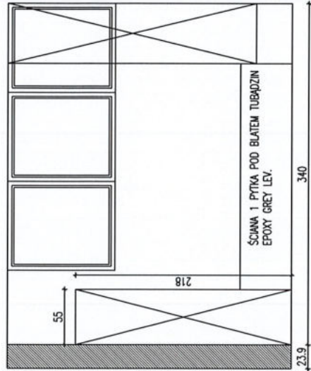
WIDOK ŚCIANY 2
